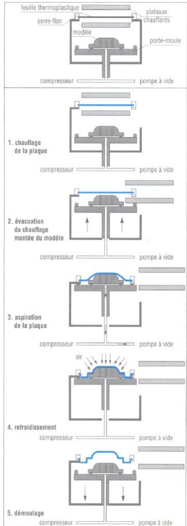
Fig. 1. Principe du thermoformage.
