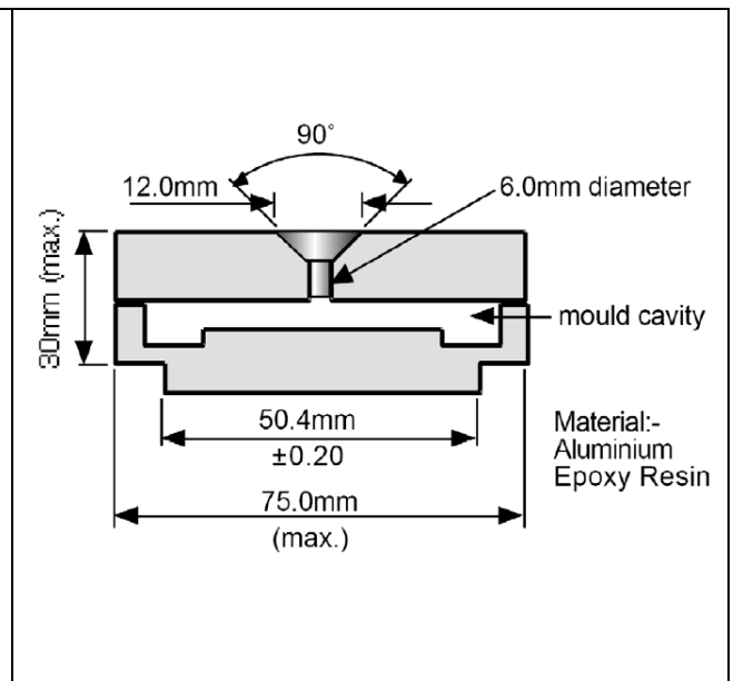
Figure 2 – Paramètres du moule.
